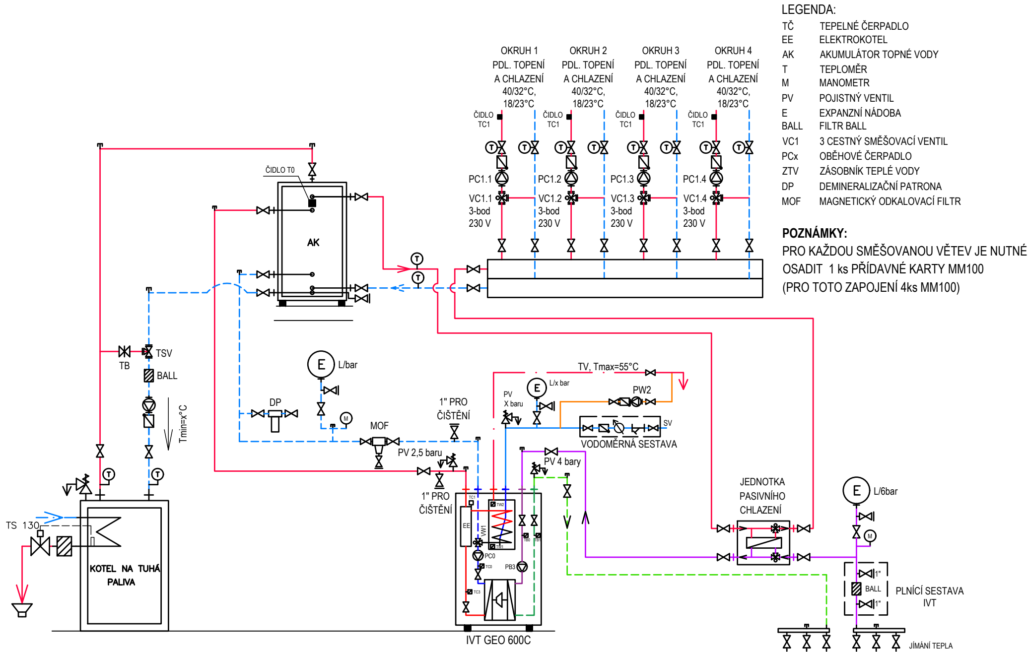
IVT GEO 600C - 4 top/chl okruhy s akumulátorem + pasivní chlazení + kotel
