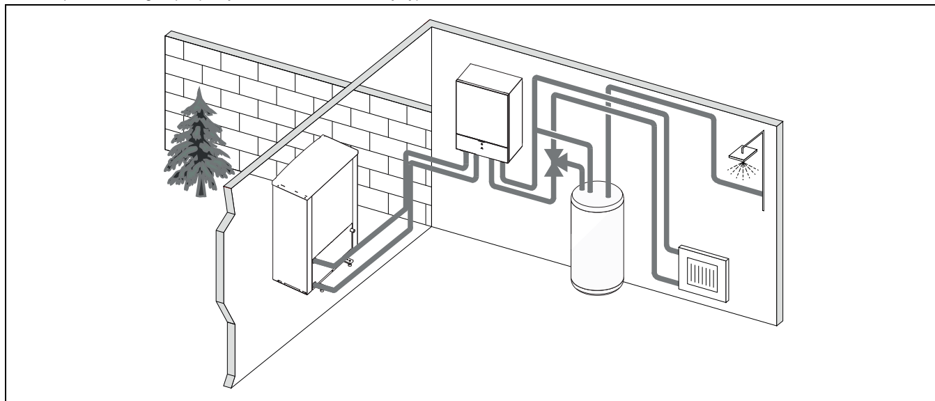
Obr. 3 Tepelné čerpadlo AirX 400, vnitřní jednotka Airbox E s elektrickou pomocnou topnou tyčí a externím zásobníkem teplé vody
